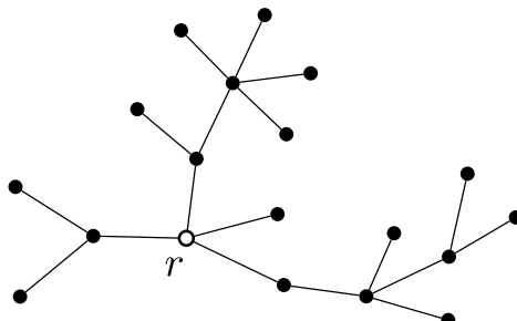
1. ábra: Egy gyökeres fa (amelyben az r csúcs a gyökér).
