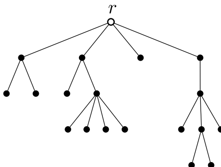
2. ábra: Az előző ábrán szereplő fa lerajzolása „családfaszerűen”.
