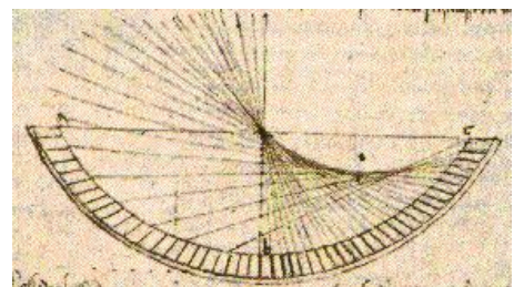
Sugarak, visszaverődés?
